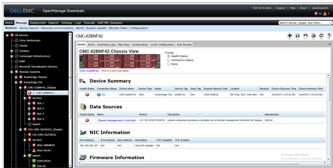
Abbildung 22. Gehäuse-Ansicht
